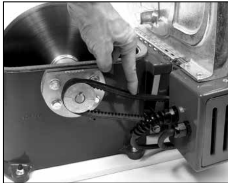
Fig. 29. Belt tension
